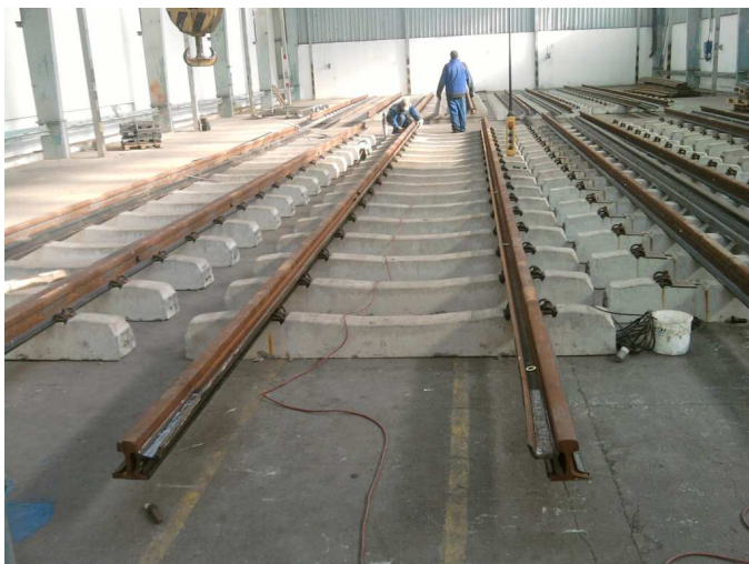
Žlábkovací profil Spurrillenschiene S49 předmontovaný v Pražské strojárně a.s. na betonové pražce a zabudovaný v Praze
