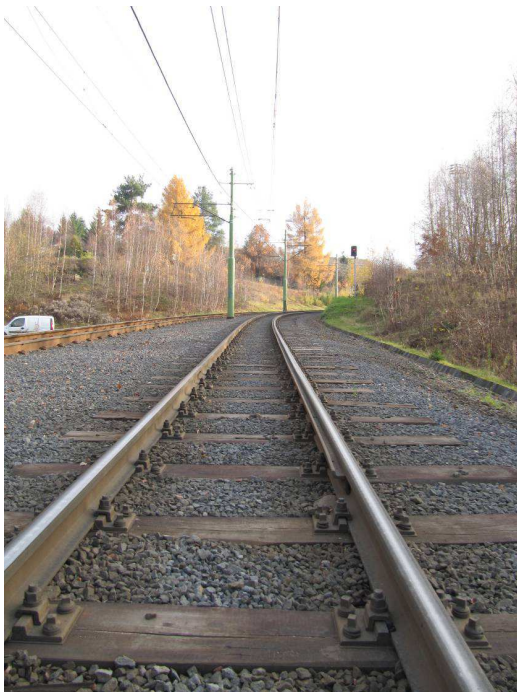
Přídržnice z profilu Spurrillenschiene S49 v oblouku v Liberci
