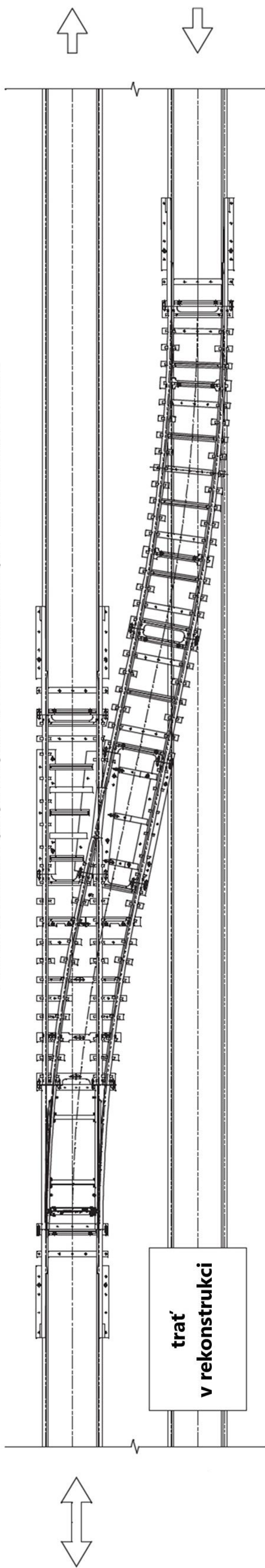
Použití mobilního přejezdu jako dočasné obratiště pro obousměrná vozidla
